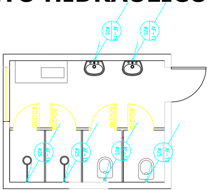
PLANTA BAIXA - BANHEIRO SALA MATERNAL ESCALA:1/50
