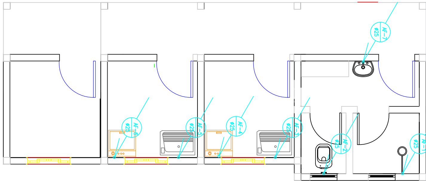
PLANTA BAIXA - VESTIÁRIO - FUNDOS CEMEI ESCALA:1/50
