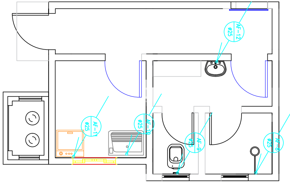
PLANTA BAIXA - VESTIÁRIO COZINHA ESCALA:1/50
