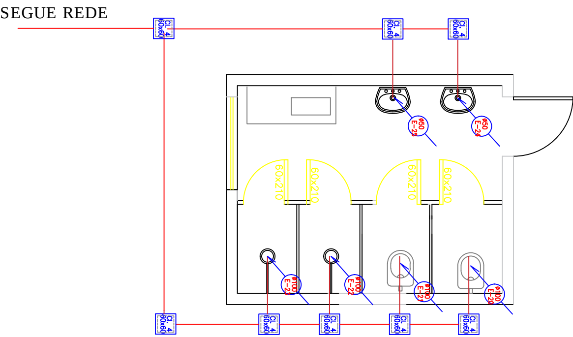
PLANTA BAIXA - BANHEIRO SALA MATERNAL ESCALA:1/50
