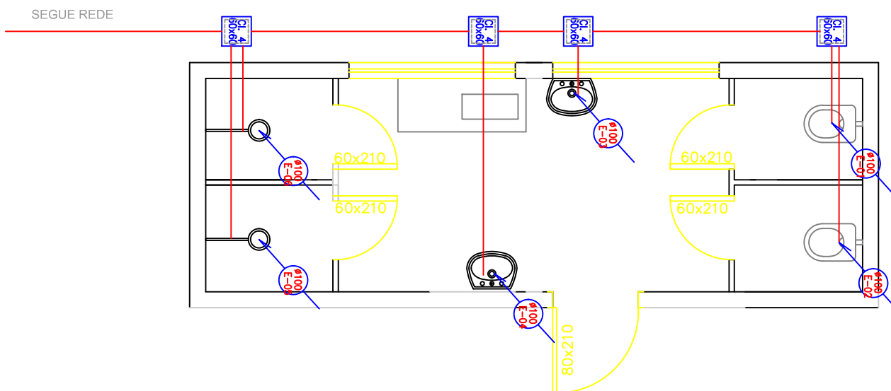
PLANTA BAIXA VESTIARIO -MATERNAL 2 ESCALA:1/50
