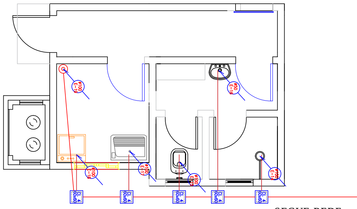
PLANTA BAIXA - VESTIÁRIO COZINHA ESCALA:1/50
