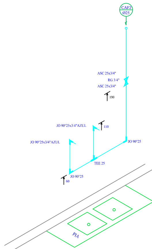
ISOMÉTRICO 04 ESC:1/25
