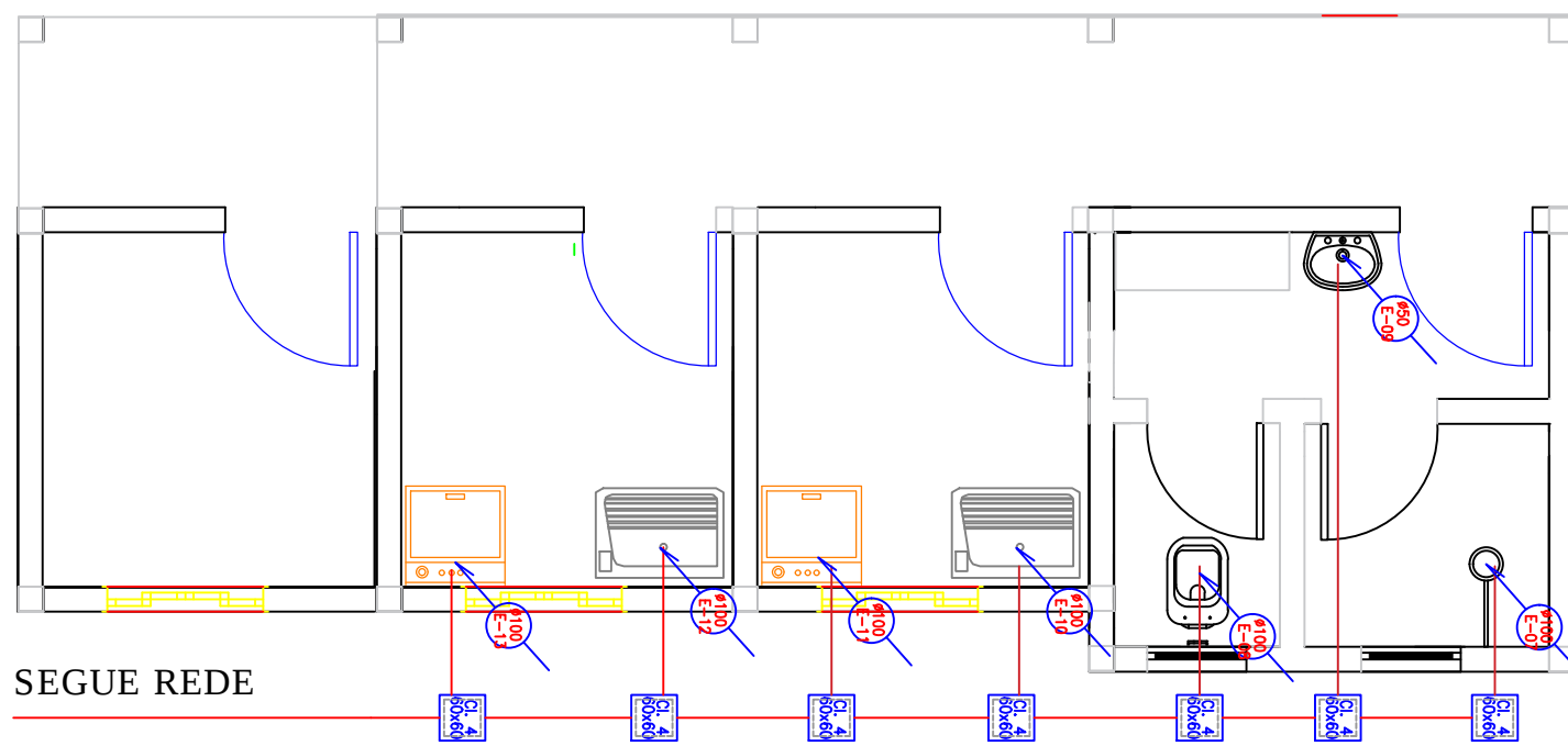
PLANTA BAIXA - VESTIÁRIO - FUNDOS CEMEI ESCALA:1/50
