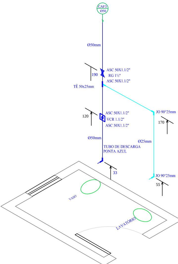
ISOMÉTRICO 03 SEM ESCALA
