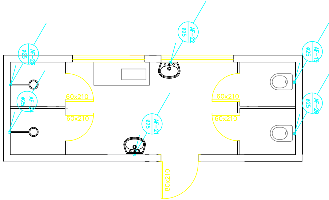
PLANTA BAIXA VESTIARIO -MATERNAL 2 ESCALA:1/50
